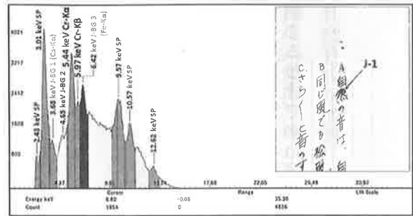
▲ペン習字浄書インクの蛍光X線分析の結果。蛍光X線がエネルギーごとにどれぐらいに発生しているかピークになってあらわれる。ピークの高さが測定された元素の数を示す。クロム元素固有の蛍光X線が発生していることがわかる。
